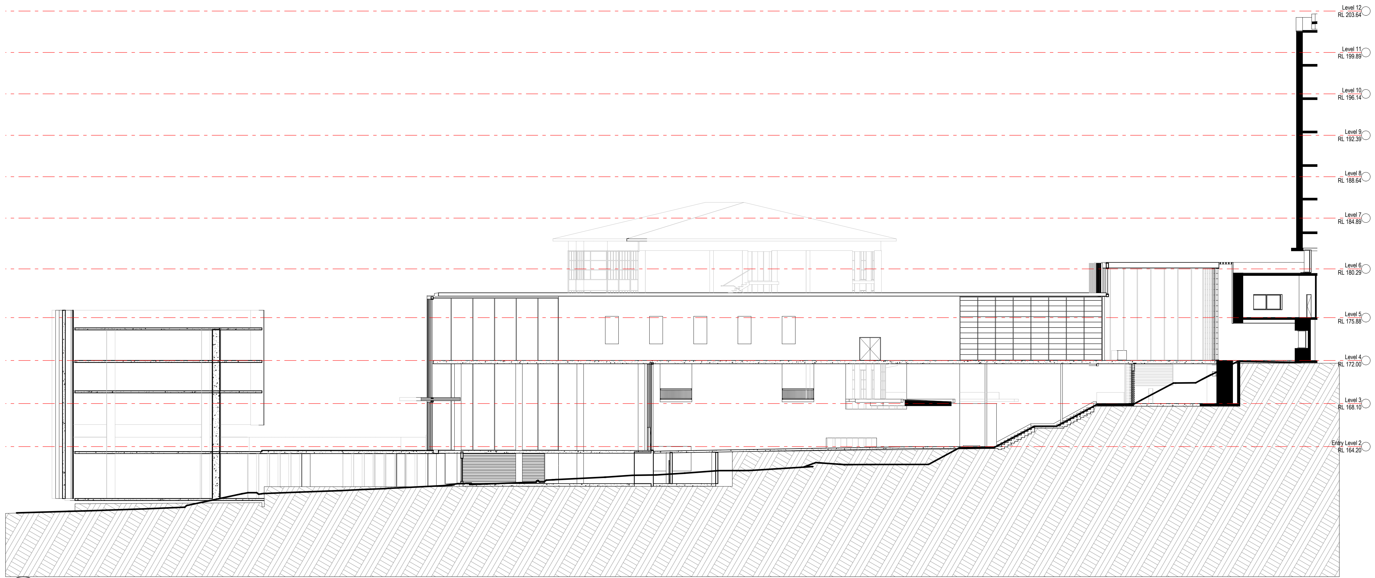
1 E-A SECTION A SCALE 1:200
